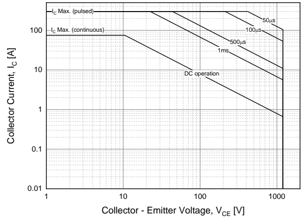
Fig. 14 SOA
