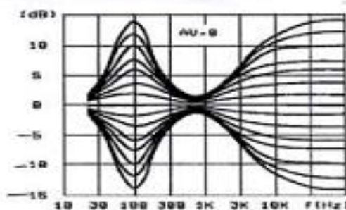
频率特性
