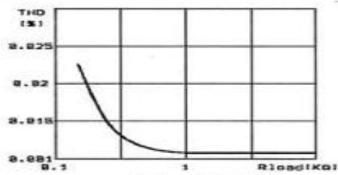
失真 vs 负载电阻
