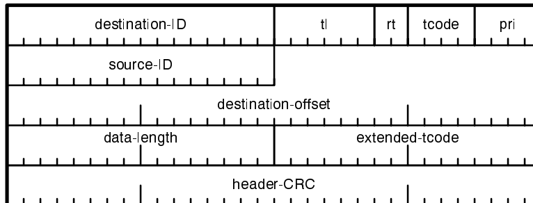
packet-format
